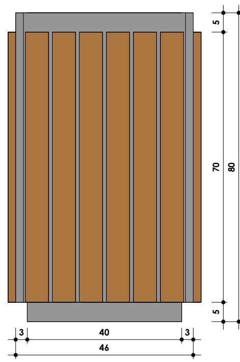
11 Elevação direita 1 : 10
