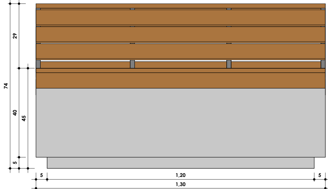
3 Elevação frontal1 1 : 10
