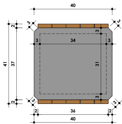
5 Elevação de topo 1 : 10
