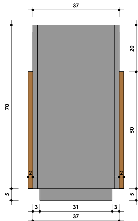
7 Elevação direita 1 : 10
