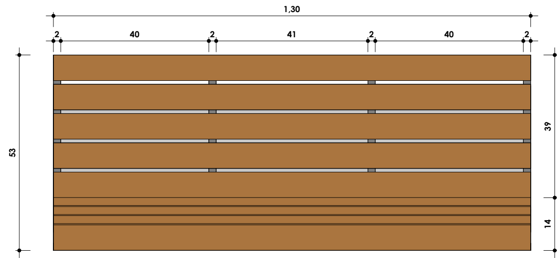
1 Elevação de topo 1 : 10
