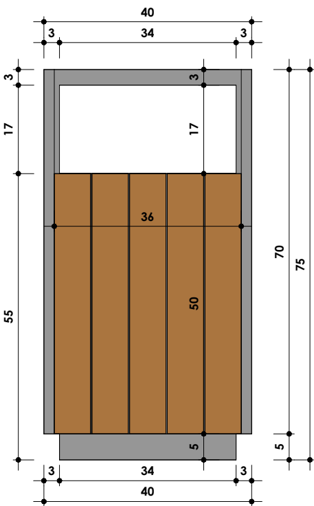
6 Elevação frontal 1 : 10
