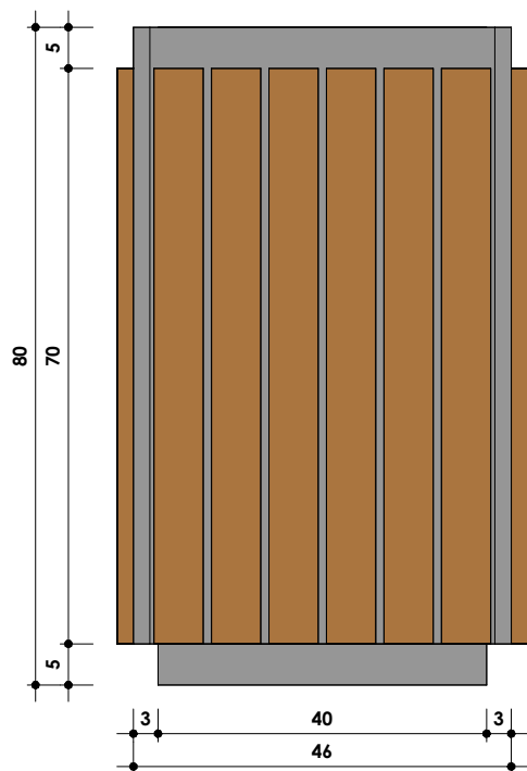
10 Elevação frontal 1 : 10
