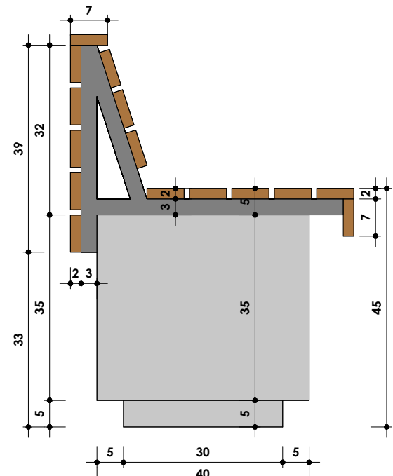
2 Elevação direita1 1 : 10
