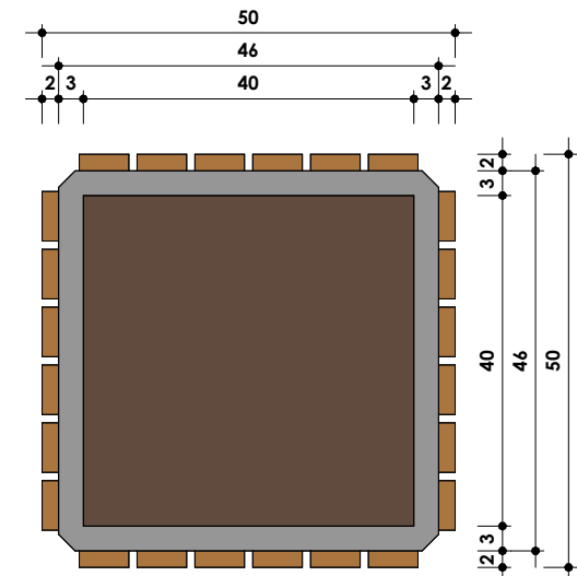
9 Elevação de topo 1 : 10
