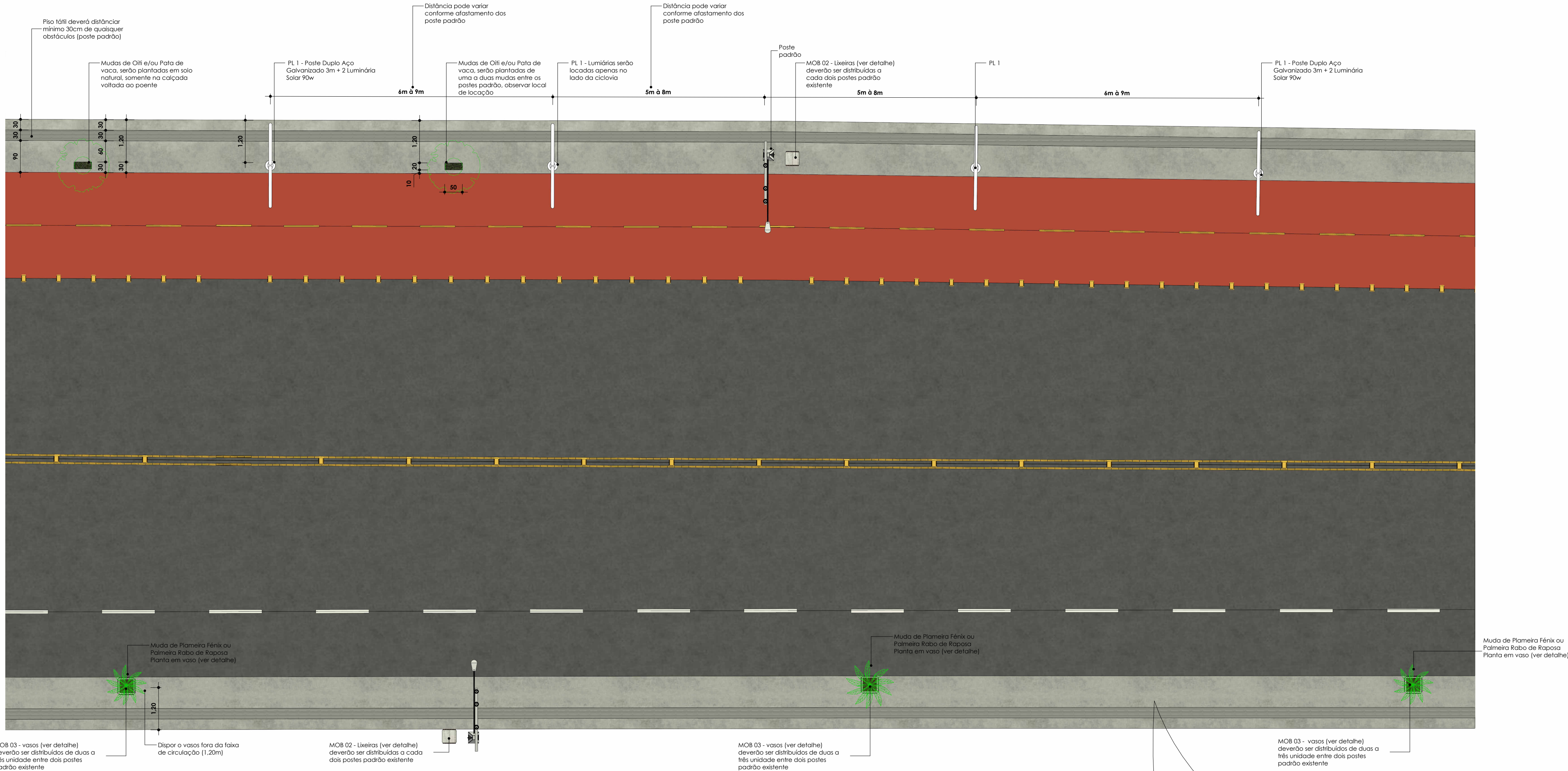
1 Planta Baixa - trecho comum 1 : 75
