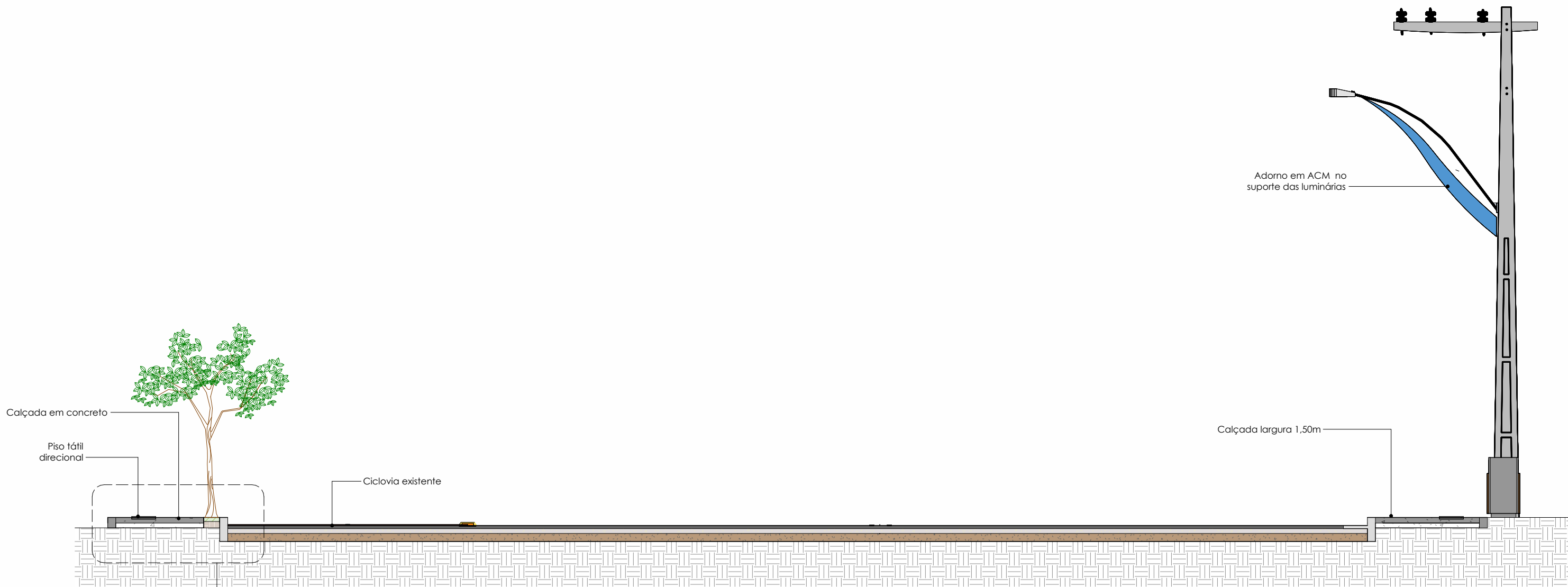
4 Corte 2 1 : 50
