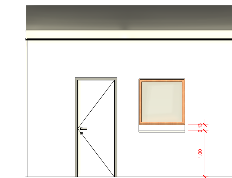
4 Corte 1 1: 50
