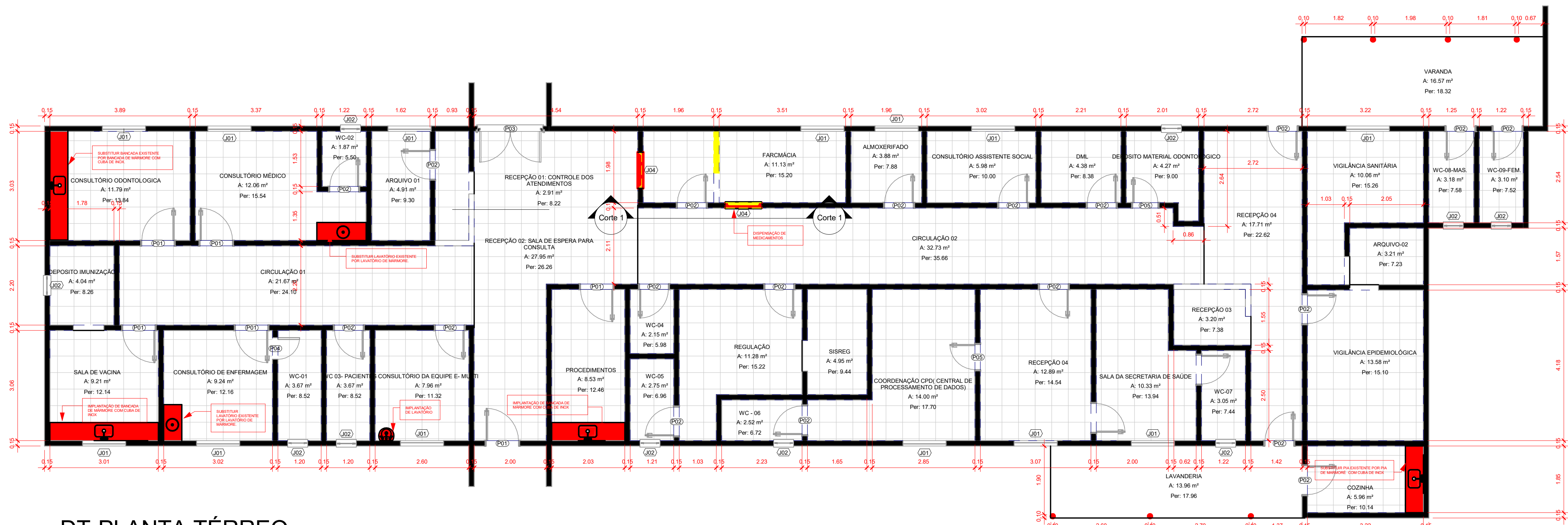
1 DT-PLANTA TÉRREO - REFORMA- COTAS 1:75
