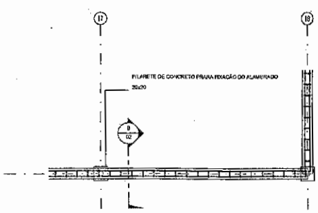
FERRAGEM NÍVEL - DET-02 ESCALA 1:20
