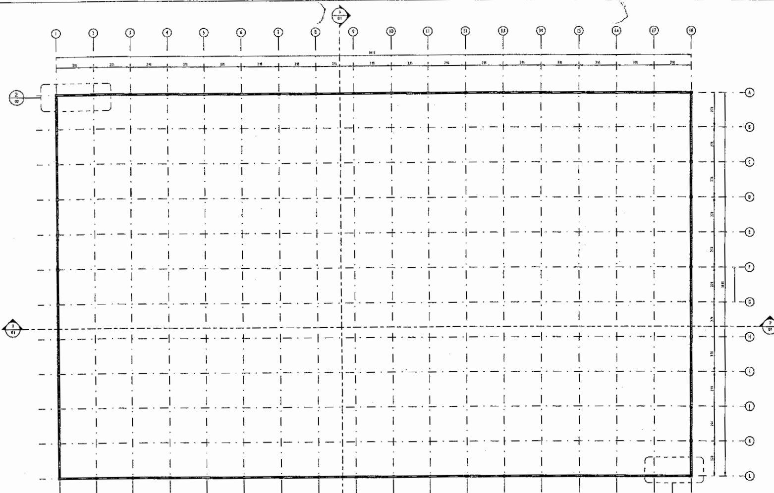
FERRAGEM NÍVEL 00 ESCALA 1:100
