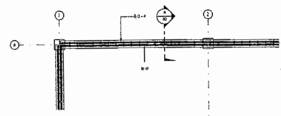
FERRAGEM NÍVEL - DET-01 ESCALA 1:20
